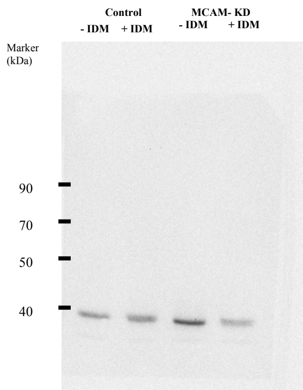
ERK2
