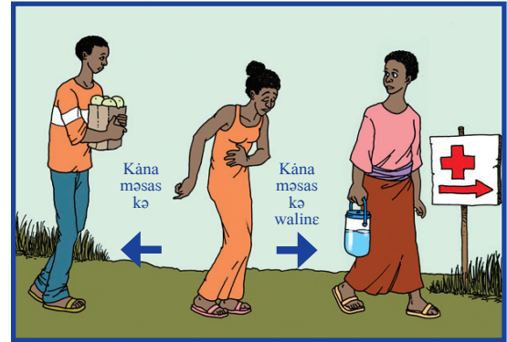
Marāne aŃbonsħo āmu
