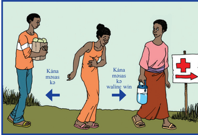
Marāne āŃbōnshō āmu
