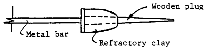
Slag Tap Hole Plug
