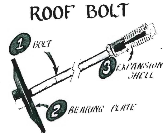
Figure 9. A roof bolt.
