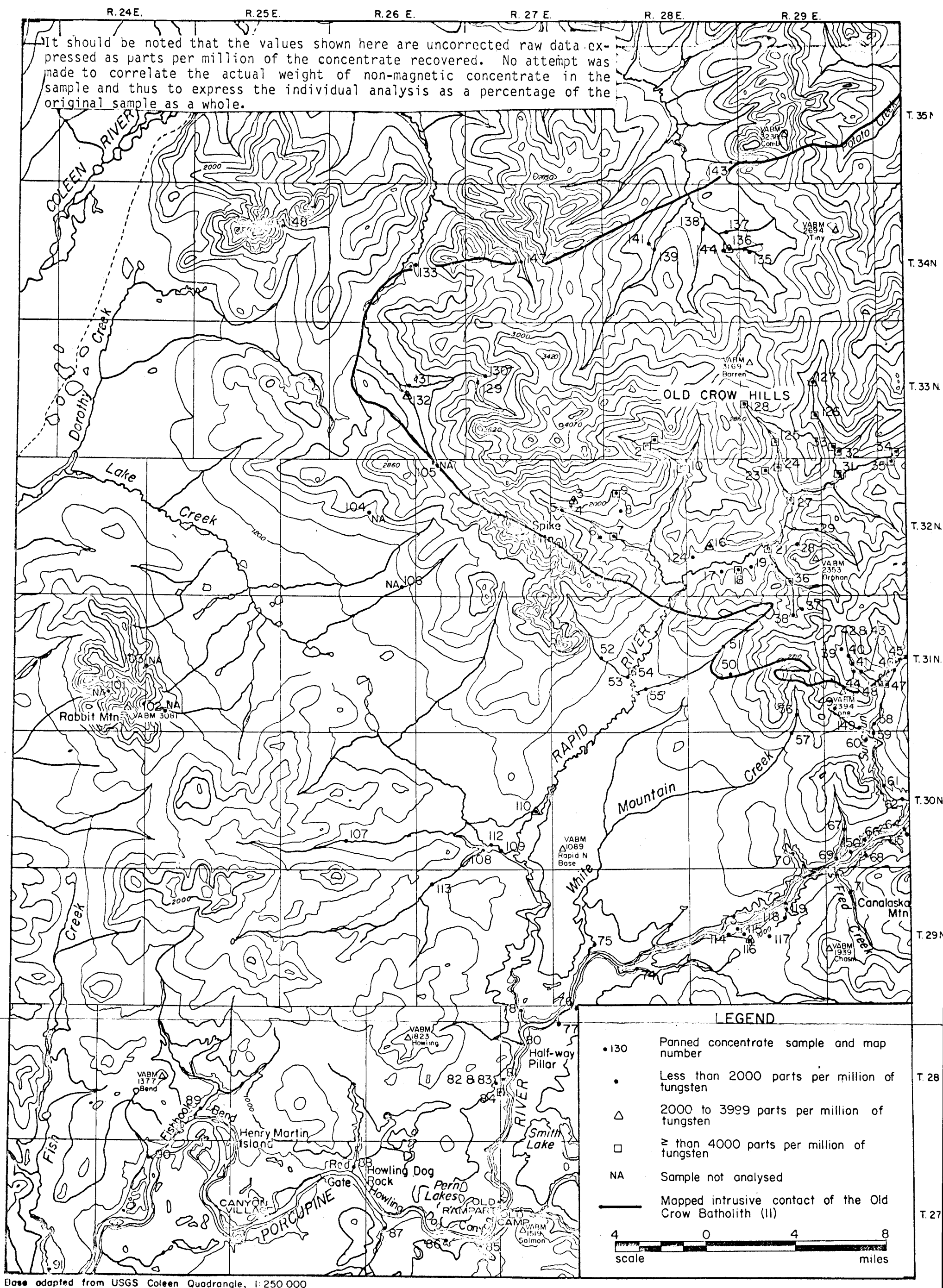
FIGURE 27.- Tungsten analyses--Old Crow Hills
