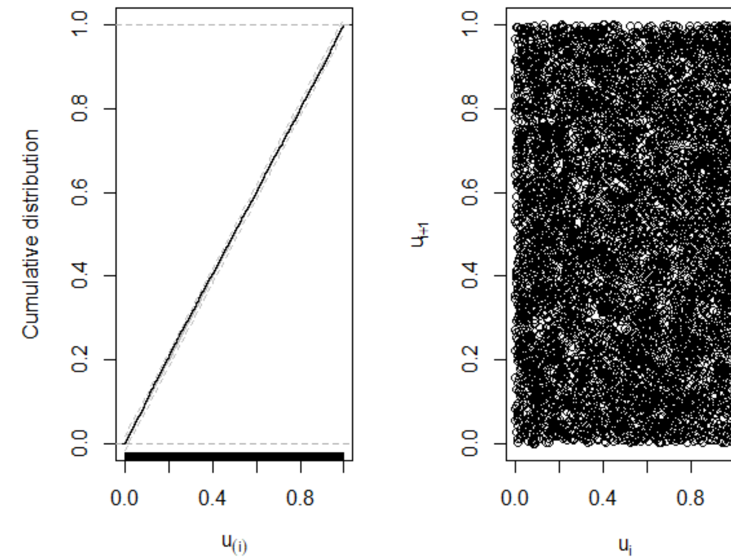
F. Twinstim model: 250 meters, 14 days
