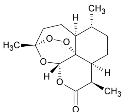
Artemisinin
