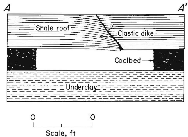
ELEVATION A-A'
